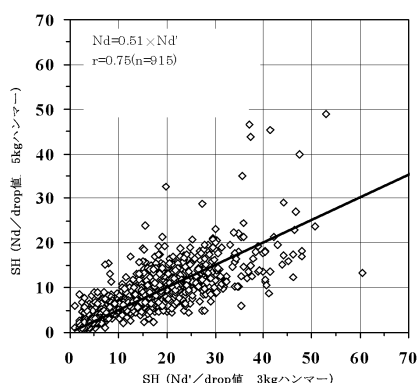
図 2.1 「Nd'/drop」と「Nd/drop」の関係
