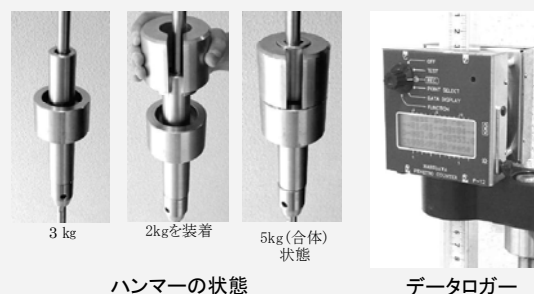
写真 1.1 ハンマーとデーターロガー
