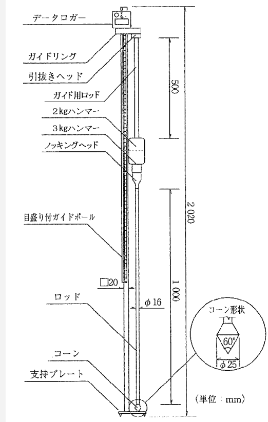
図 1.1 SH型貫入試験機
